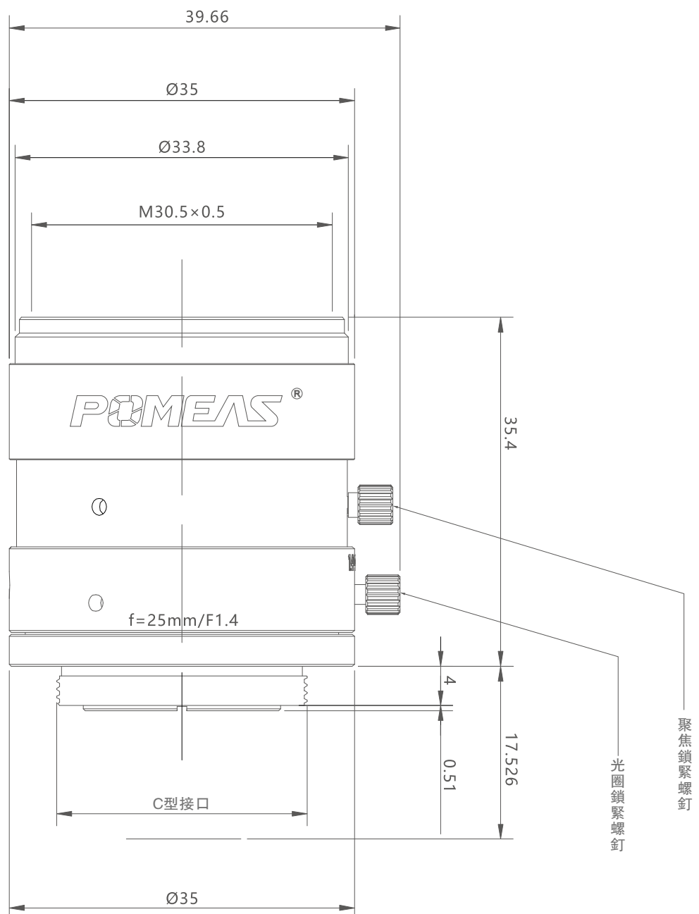
產品尺寸圖
