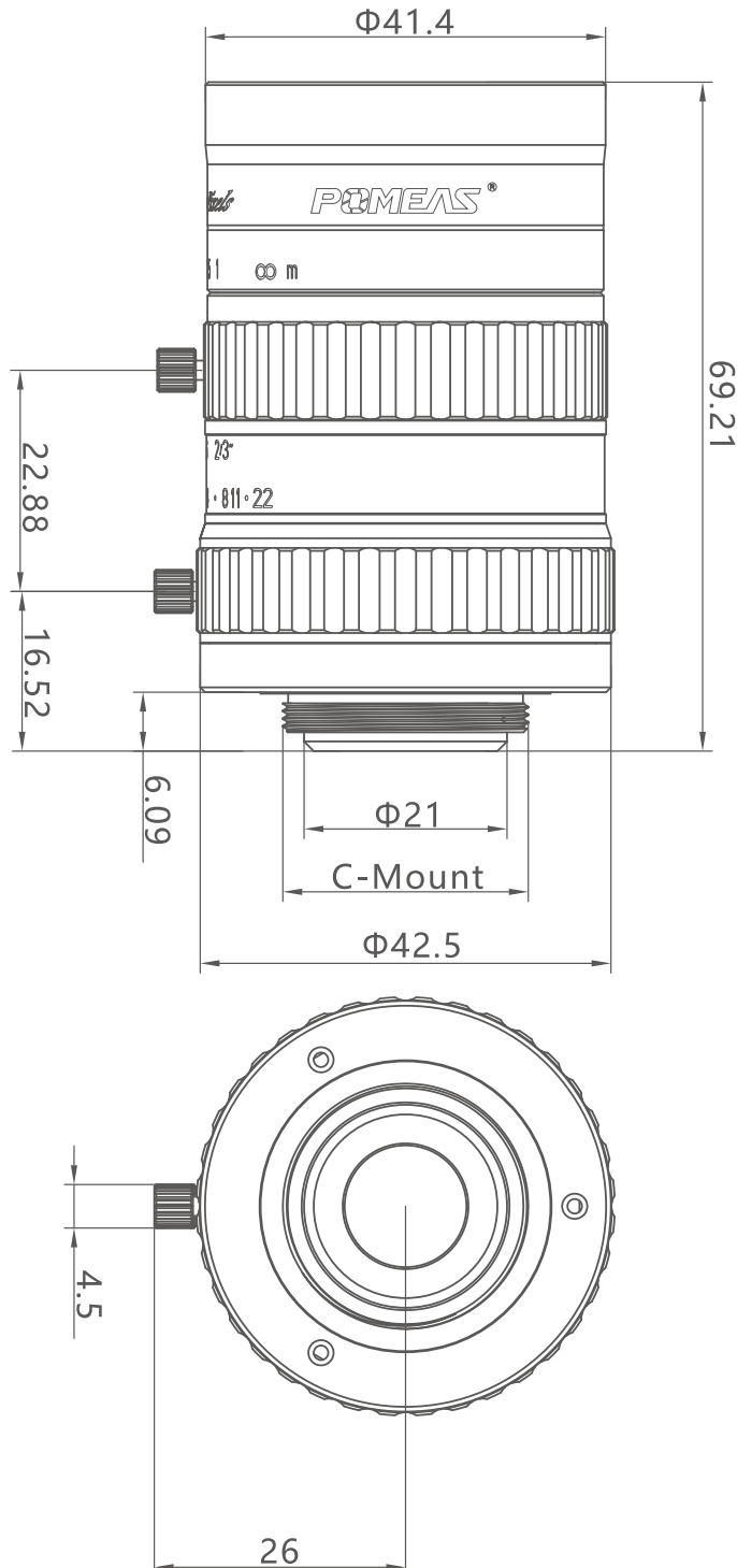
產品尺寸圖
